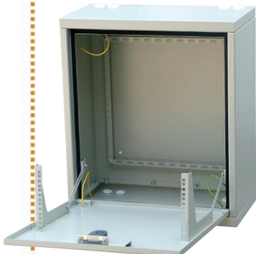
Рисунок 2: Дверные кронштейны
