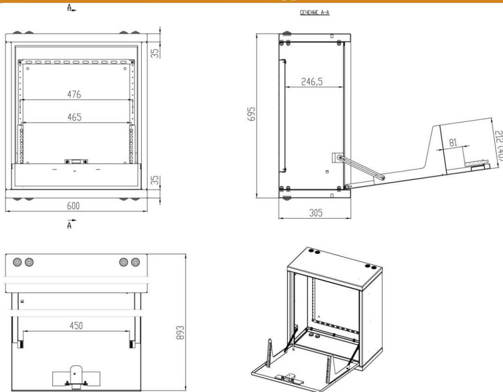
Рисунок 4: Монтажно-габаритные чертежи
